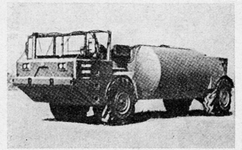
Bild 2. «Goer»-Tankfahrzeug
