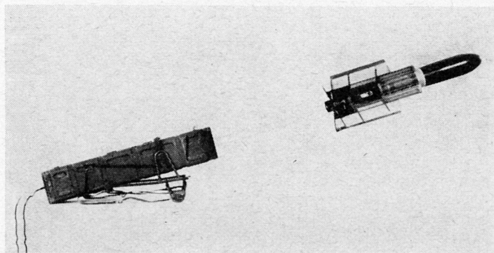
Abschuß der Lenkwaffe aus dem Startbehälter.
