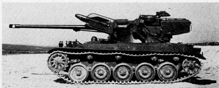
Auf dem Leichtpanzer AMX montierte Abschußrampen für vier SS 11. Die mit dem 105-mm-Geschütz und mit vier SS 11-Abschußrampen ausgerüsteten AMX finden in den französischen Panzerjägerverbänden Verwendung.
