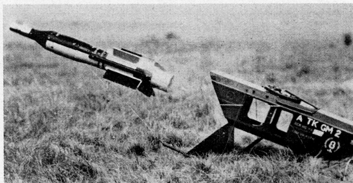
Abschuß der Lenkwaffe aus dem Startbehälter (älteres Modell der Lenkwaffe).
