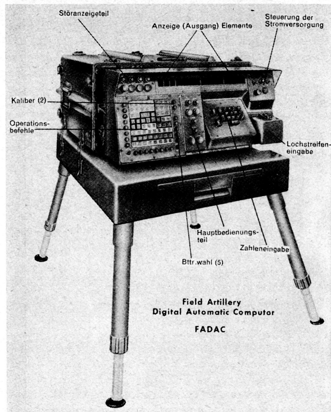
Bild 4. Gesamtansicht FADAC.
