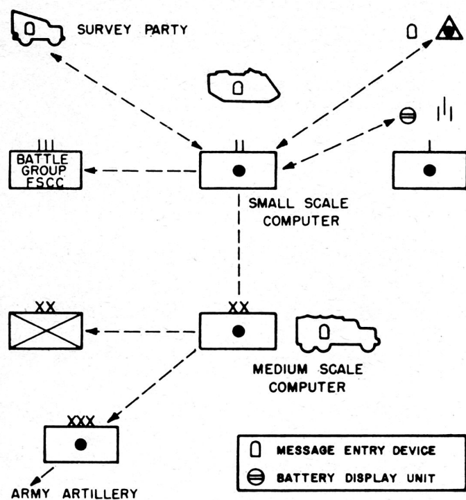
Bild 3. Aufbau Feuerleitteilsystem.
