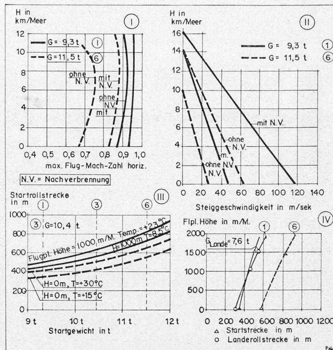
Figur 2. Kurze Übersicht auf wesentliche Flugleistungen, wie:
