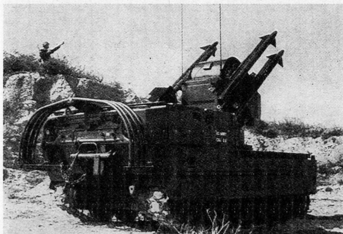
Bild 12. Prototyp XM 548 «Chaparral» (USA). Amerikanische Notlösung mit der bewährten Rakete «Sidewinder», die einen aktiven Infrarotsuchkopf hat; Fahrgestell des Schützenpanzers M 113; Abschub-turm ungepanzert.
