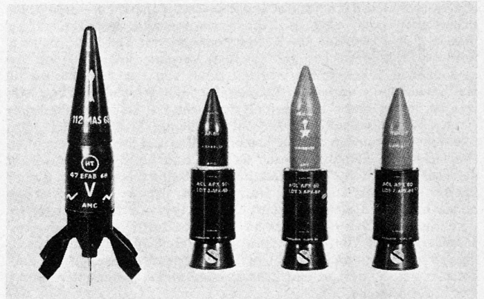
Bild 2. Das Geschöß mit Hohlladungsgefechtskopf und ausgeklappten Stabilisierungsflächen. Neben Hohlladungsgeschossen kann die Panzerfaust auch andere Munition zum Einsatz bringen; von links nach rechts: Spreng/Splitter-Munition, Leuchtmunition, Nebelmunition.
