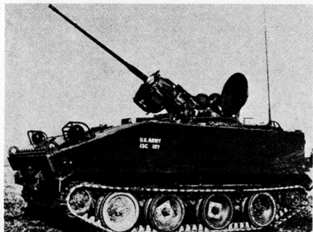
Bild 1. Der Spähpanzer M114 AI (leichter Spähtrupp).
