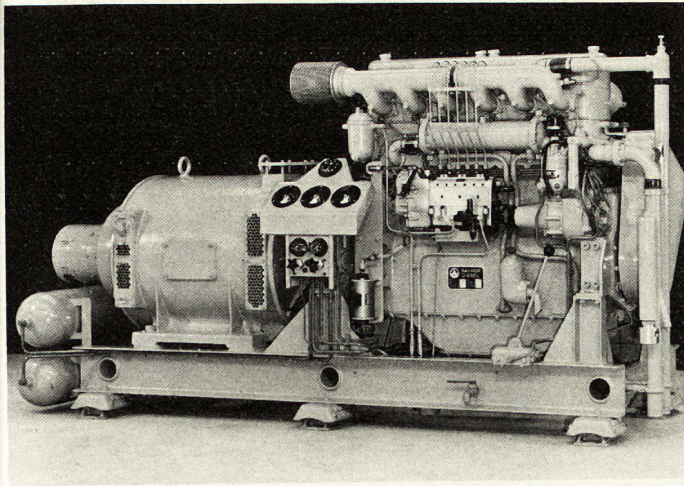
Saurer-Notstromanlage, 180 PS, mit BXD-Motor, auf Gummi-Metallsockeln gelagert.
