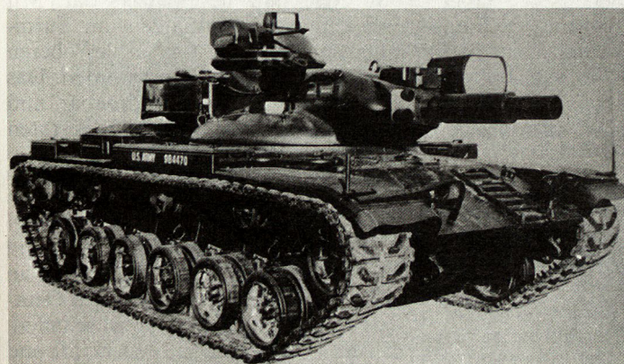
Bild 4. Der amerikanische M60 A2 mit der 152-mm-Kombinationswaffe.
