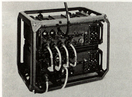
Fig. 5. Beispiel eines MK-7-Gerätes mit Schwingrahmen.
