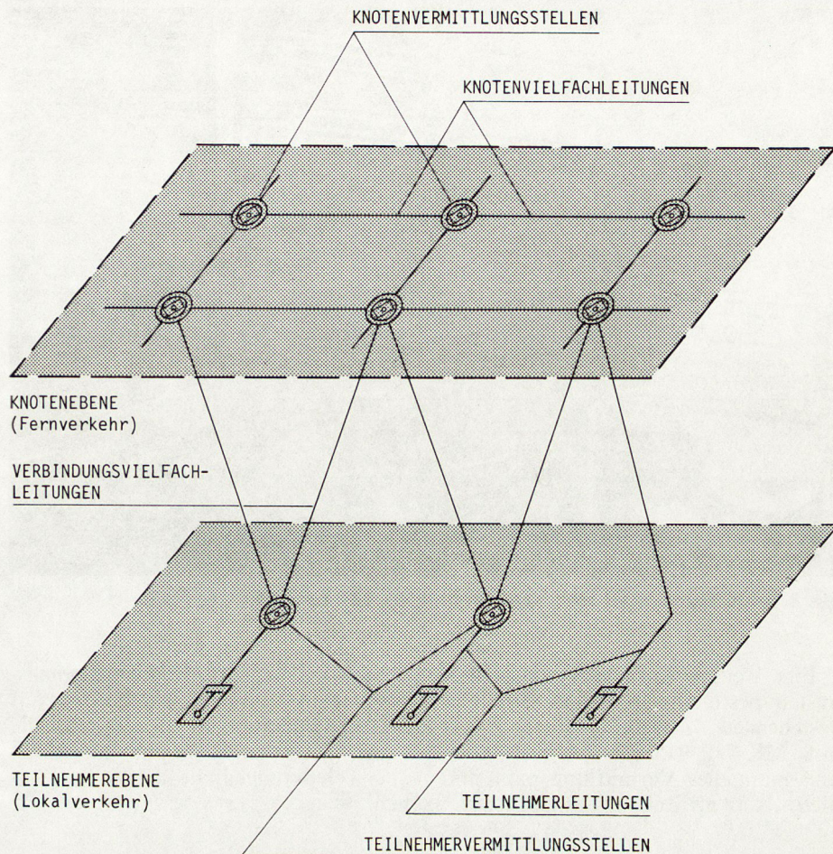
Fig. 6. Mögliche IBEX-Netzstruktur.
