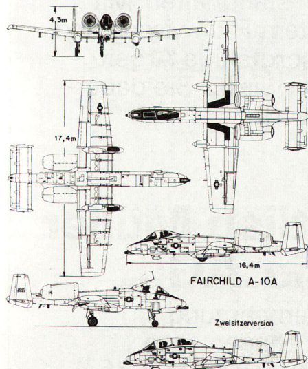
Bild 1. Kampfflugzeug Fairchild A 10 A.
