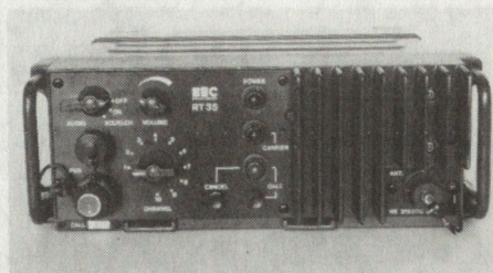
Bild 2. Der «Securadio 35» ist ein Mobilfunkgerät in Militärausführung, ebenfalls mit eingebauter Sprachverschlüsselung. (Bild BBC)
