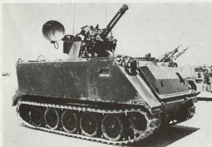
Bild 24. «Vulcan» 20-mm-Gatling:
