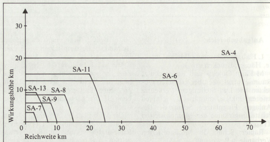
Bild 1. Lenkwaffen-Fliegerabwehrschirm Ost
