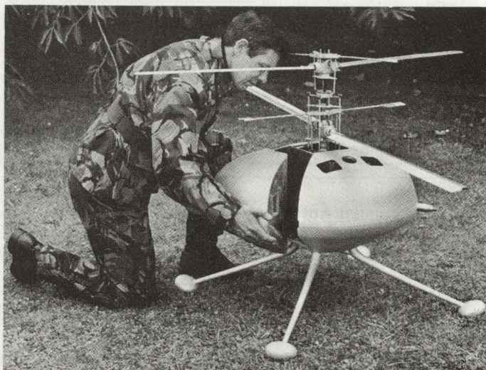
Bild 4: RPH, Kleindrohne «Sprite» (Loral), der 2. Generation, die für die Divisionsstufe in Frage kommt.
