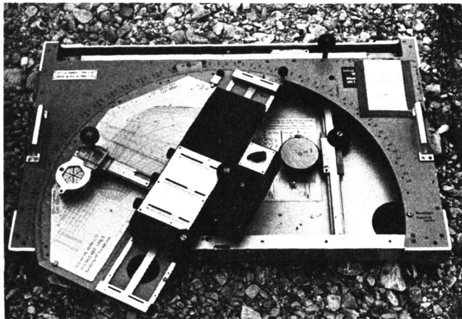
Bild 19. Schiesserelementrechner (SER)
