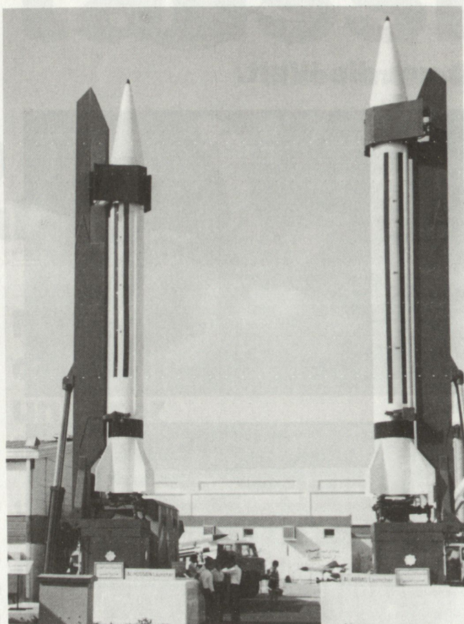
Ausstellung der irakischen Boden-Boden-Lenk Waffen Al Hussein in Bagdad.
