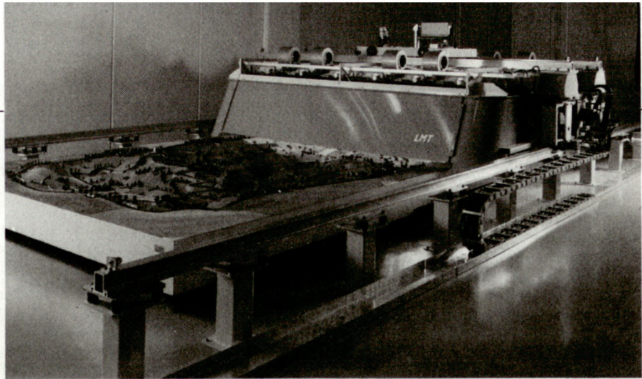
Geländemodell als Bestandteil eines Panzer-Fahrsimulators (Leo 2) auf dem Waffenplatz Thun (Armee fotodienst)
