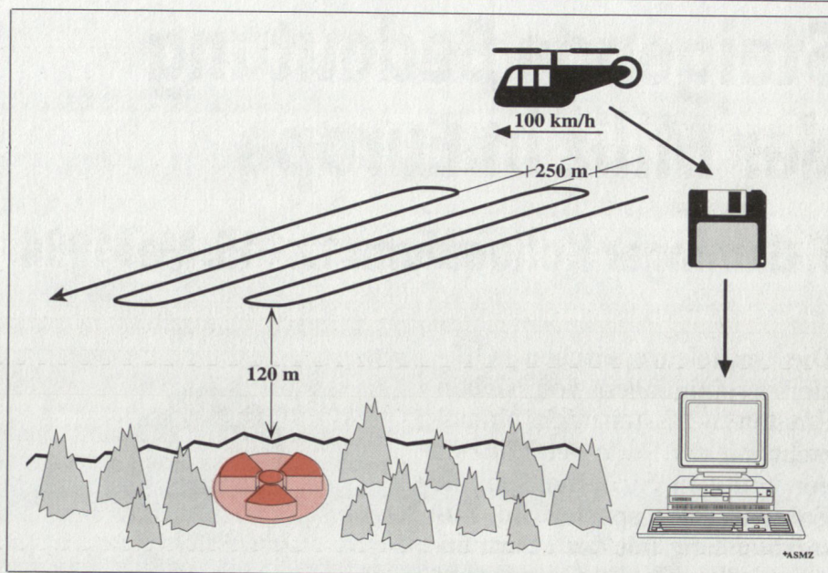
Flugtaktik beim Ausmessen einer Bodenverstrahlung und bei der Suche nach einer Strahlenquelle.
