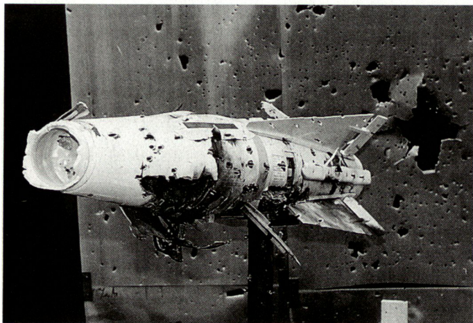
Abb. 3: Nicht mehr flugfähig: Mit AHEAD-Munition beschossene «Falcon»-Rakete. Die im Hintergrund sichtbaren, 3 mm dicken Aluminium-Kontrollplatten zeigen die Streuung der Subprojektil auf.
