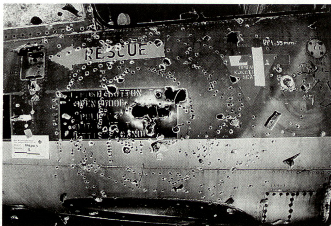
Abb. 4: Der mit AHEAD-Munition beschossene Rumpf einer F-104 belegt eindrücklich die verheerenden Auswirkungen der Wolfram-Subprojektil. (Aufnahmen: Oerlikon-Contraves)
