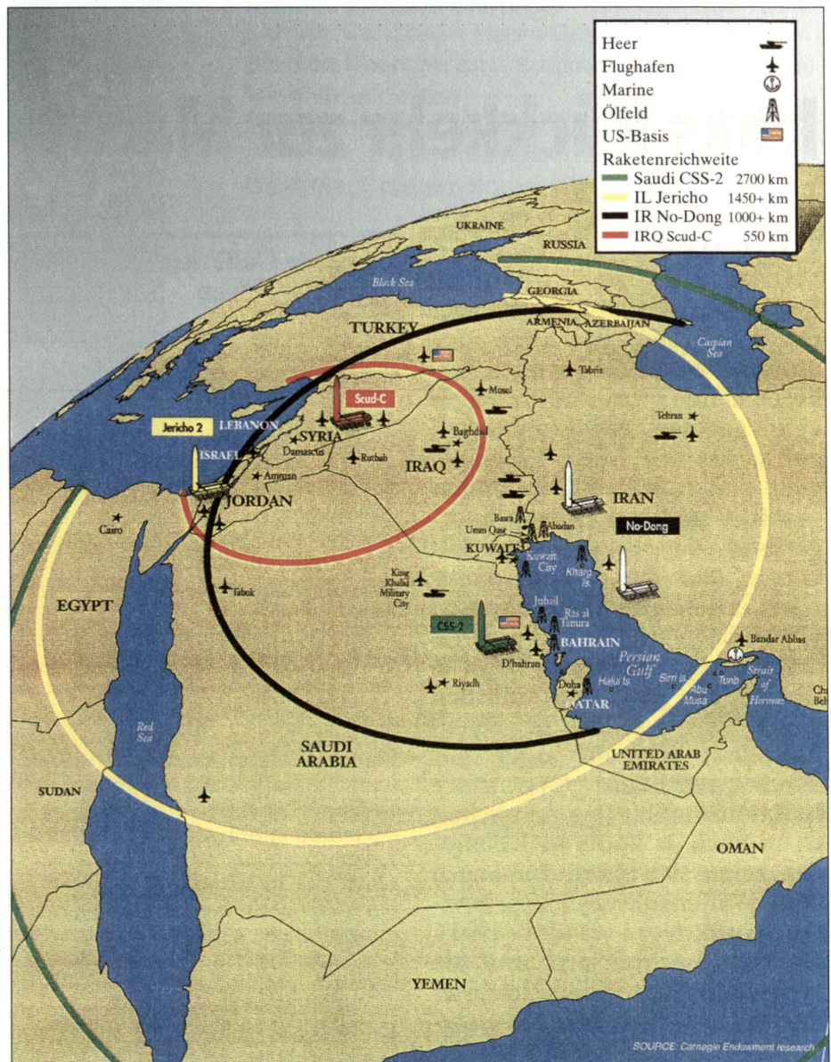
Raketenreichweiten der Nahost-Staaten.
