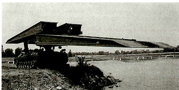
Panzerschnellbrücke «Biber».
