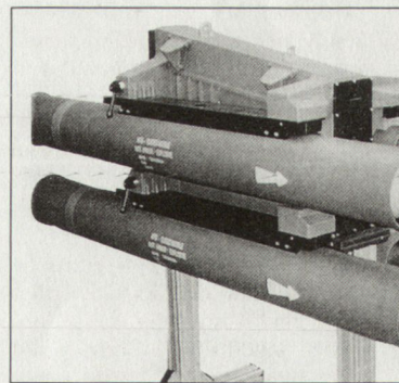
Abschusscontainer für die helikopterstützte Waffe «NTD-Dandy».
