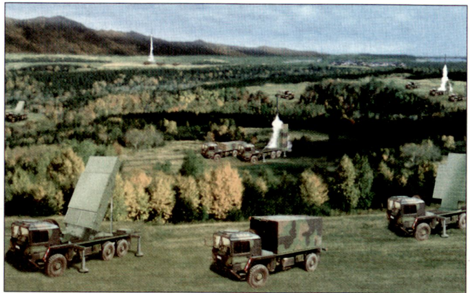
Komponenten des neuen Luftverteidigungssystems «MEADS».
