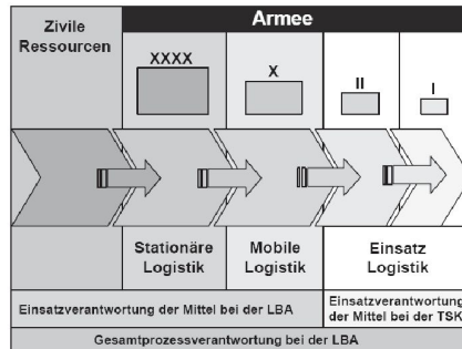
Abbildung: Ebenenmodell.
