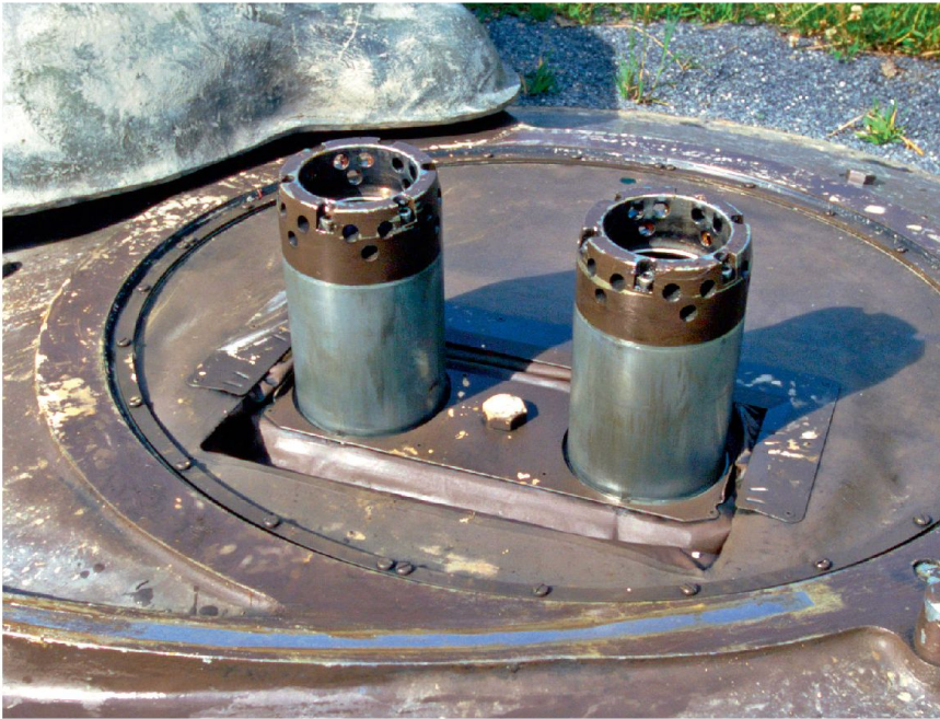
Festungsminenwerfer in offener Feuerstellung.
