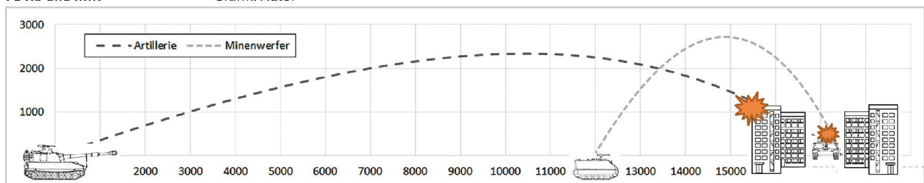
Typische Flugbahnen
