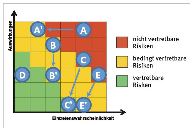
Abb. 5: Risikoraster
