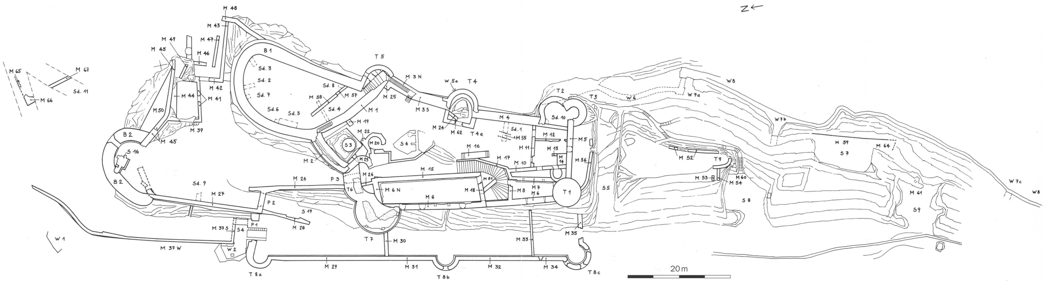
Abb. 1b Dornach, Ruine Dorneck. Gesamtgrundriss, Mst. 1:500.
