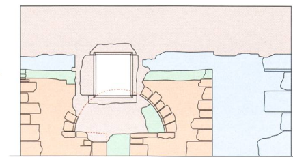
Nordfassade
