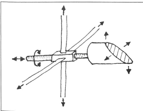
Abb. 1: Die zur exakten Einmichtung des Fangspiegels nötigen Verstellmöglichkeiten.
