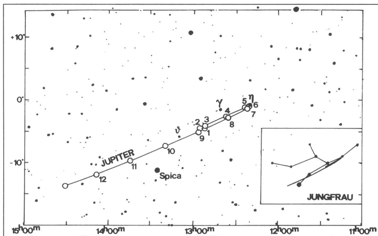
Abb. 1: Im kleinen «Fenster» ist die scheinbare Lage der Jupiterbahn im Sternbild der Jungfrau eingetragen. Der hellste Stern ist Spica. In der Ausschnittvergrösserung sind Objekte bis 10. Helligkeitsklasse dargestellt.
