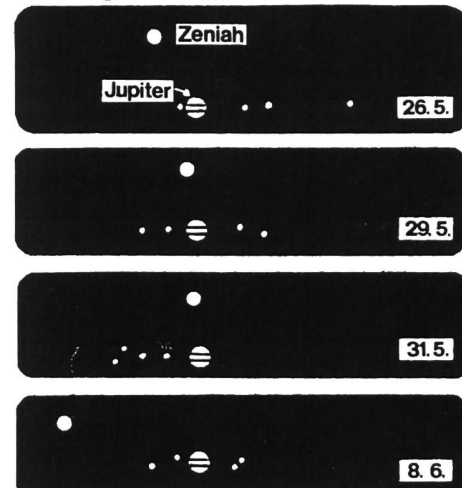
Abb. 4: Einige Situationen der Galileischen Monden mit ihrem «Fremdling» \eta Virginis.
