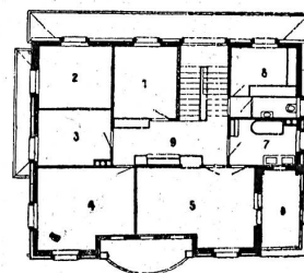
Premier étage
