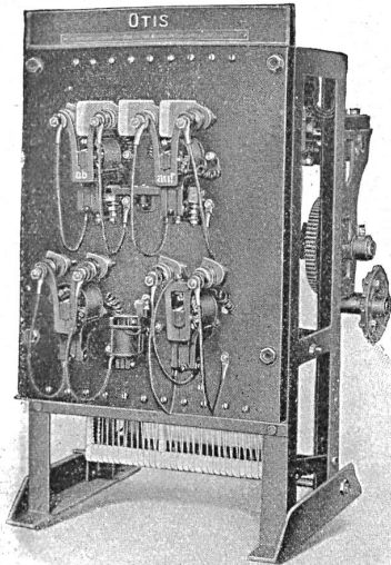
Controlleur magnétique
