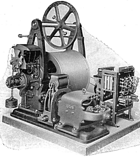
Machine d'un ascenseur pour personnes
