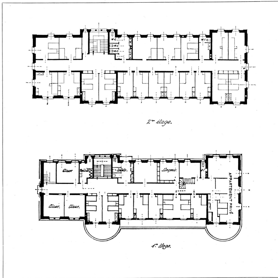
Institut de jeunes gens « La Chablière » près Lausanne. Plans du 1 er et du 2 me étages. Architecte: Georges Epiteaux, Lausanne.
