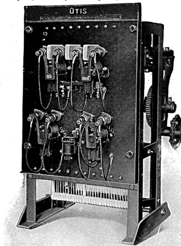
Controlleur magnétique
