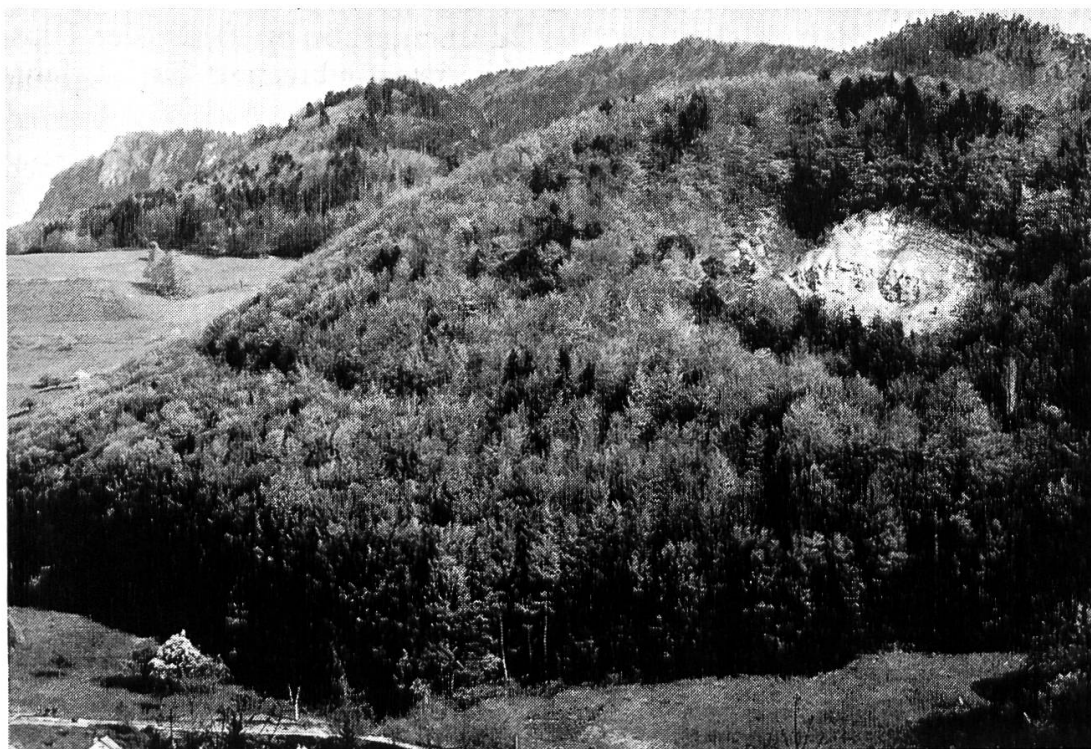
Edlisberg bei Oberdorf mit Gipsgrube von Nordosten, daneben links Riedberg, im Hintergrund von links nach rechts: Lauchflue (1041.7 m), Rehhaggrat bis und mit Breiti Flue.
