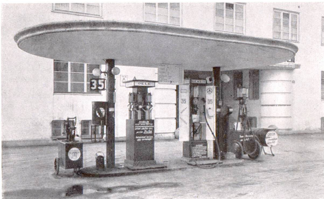
Fig. 2 Station de distribution d'essence des ateliers de réparation d'automobiles „Orion“ à Zurich. Projet: Prof. Dunkel et Ing. E. H. Nobel, Zurich Calcul: Ingénieurs Klinke et Meyer, Zurich. Exécution: Baur et Cie., S. A., Zurich
