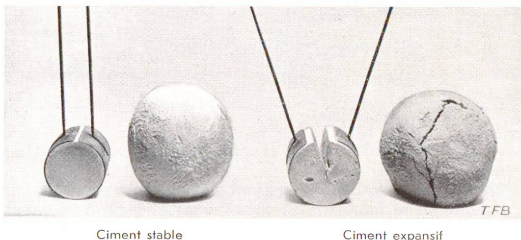
Fig. 1 Essais de laboratoire pour déterminer la stabilité des ciments.
