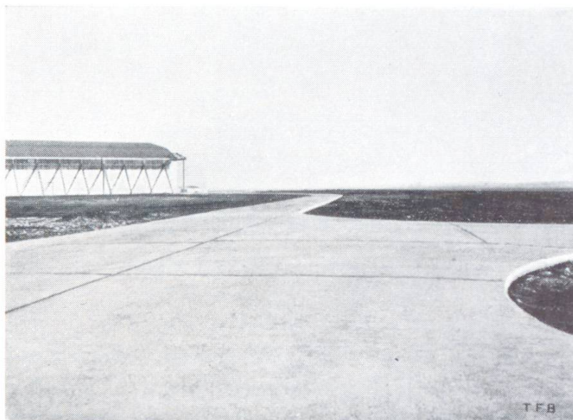
Pistes de roulement de l'aérodrome de Châteaudun, France, exécutées en béton Soliditit
