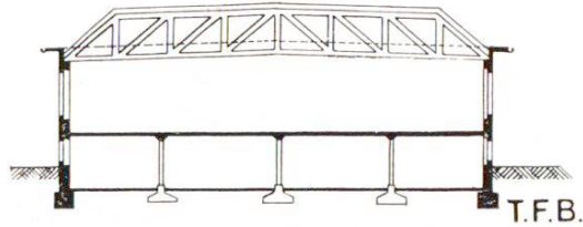
Fig. 3 Coupe longitudinale 1:250
