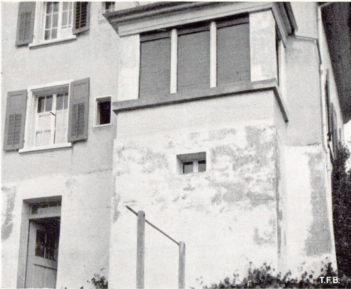
Fig. 1 Ecaillage d'une peinture à la chaux sur une fondation en béton et sur des enduits exposés
