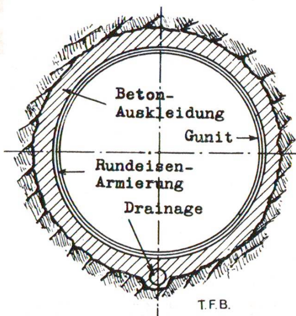
Fig. 3 Revêtement de béton avec carapace de gunit armée Fig. 4 Revêtement cuirassé
