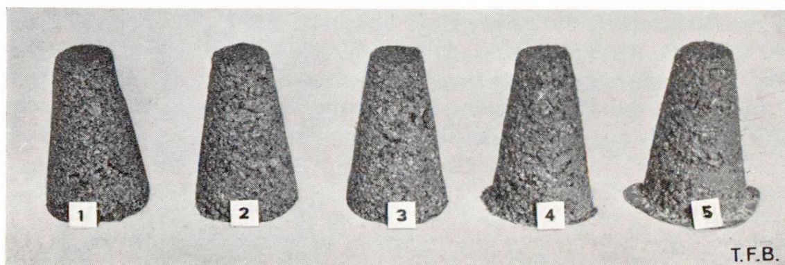
Fig. 4 L'essai d'affaissement d'un mélange dur ne révèle pas les variations de sa teneur en eau. Dans l'échantillon le plus mouillé, à droite, le mortier coule hors de l'osature des gros éléments.
