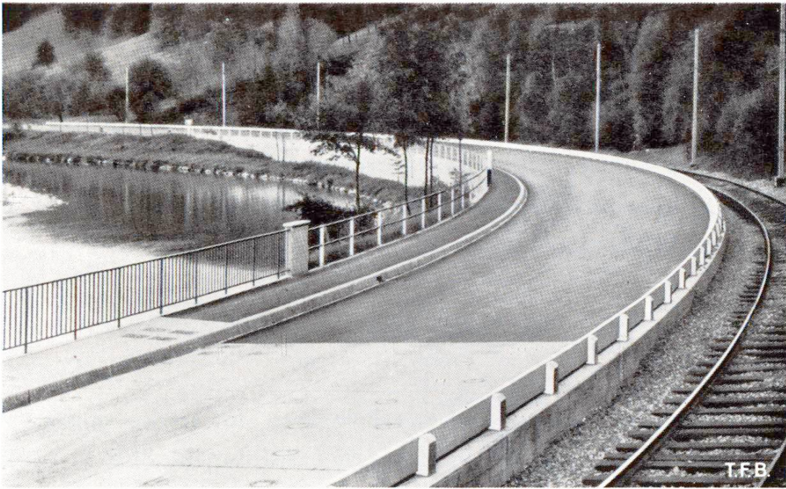
Fig. 8 Bordure de sécurité en éléments de béton préfabriqués, faciles à poser. (système suisse)
