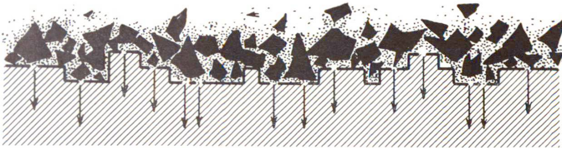
Fig. 1 Représentation schématique de l'adhérence par assemblage à dents. Le gel que produisent les grains de ciment (pointillé), très onctueux au début, entre en contact étroit avec les irrégularités de la surface du coffrage, surtout s'il s'agit d'un matériau poreux qui étant sec absorbe l'eau du béton.
