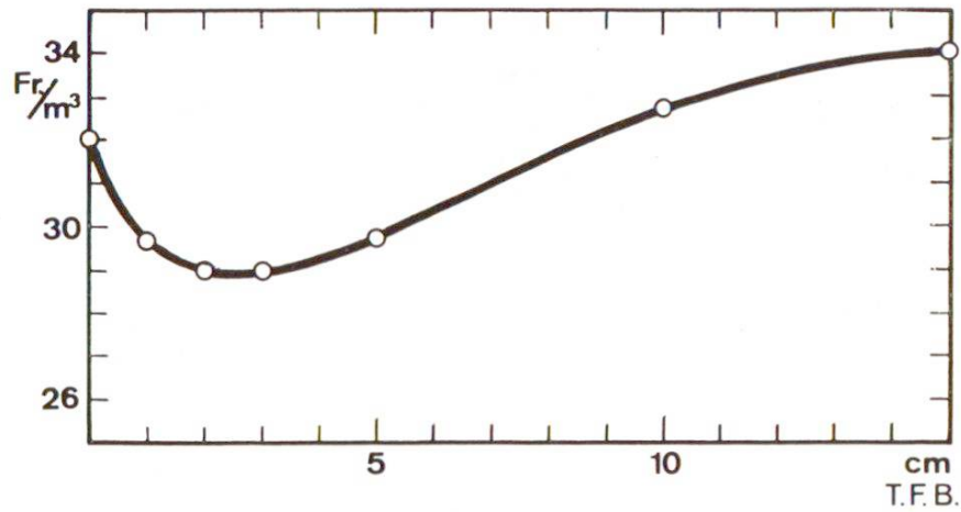
Fig. 3 Coût total du travail de mise en œuvre et du ciment en fonction de la consistance, la qualité du béton restant la même. Cette courbe est construite à partir du tableau 2 résumant les valeurs des exemples des figures 1 et 2. On constate dans ce cas un prix minimum pour un affaissement de 2-3 cm correspondant à un dosage en ciment de 285-300 kg/m 3 .
