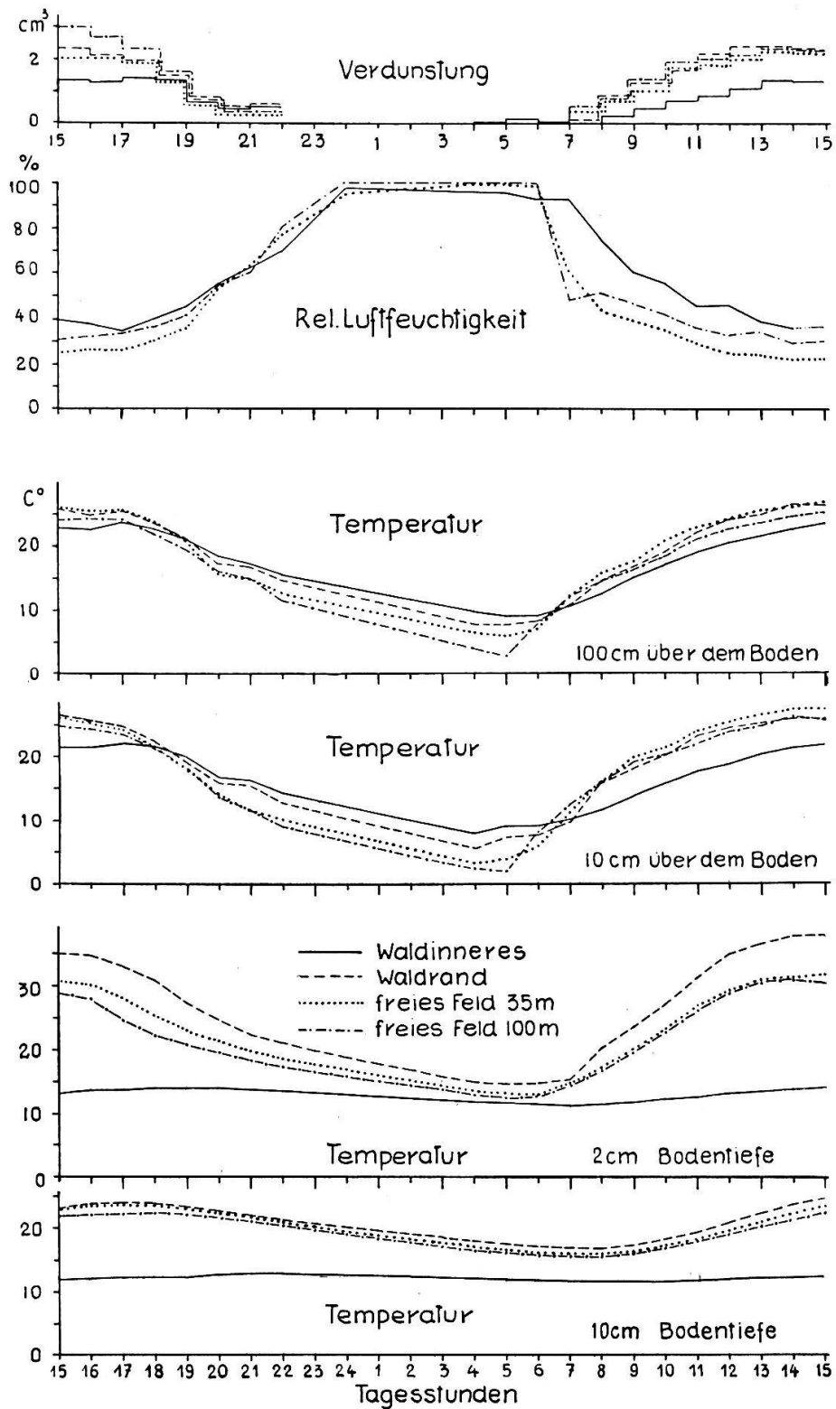
Abb. 1. Graphische Darstellung der Ergebnisse der Beobachtungen vom 18./19. Mai 1943. Bei der Luftfeuchtigkeit ist die Station Waldrand weggelassen worden, da ein Teil der Messungen nicht einwandfrei ist.
