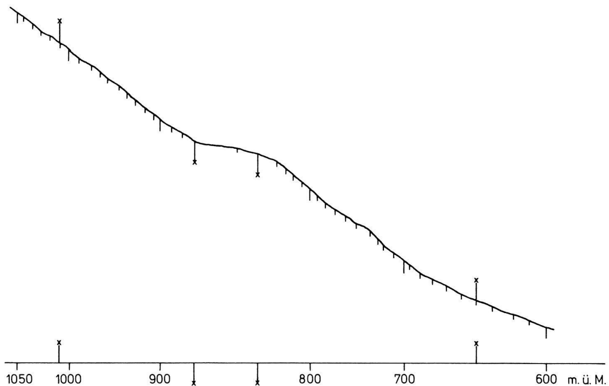
Abb. 2. Hangneigung des westlichen Profils, nach den Höhengichtlinien auf der topographischen Landeskarte der Schweiz, 1:25000, Blatt 1325 (Sembrancher), von Franz Grünweis erstellt. Die Kreuze (x) markieren Wege.
